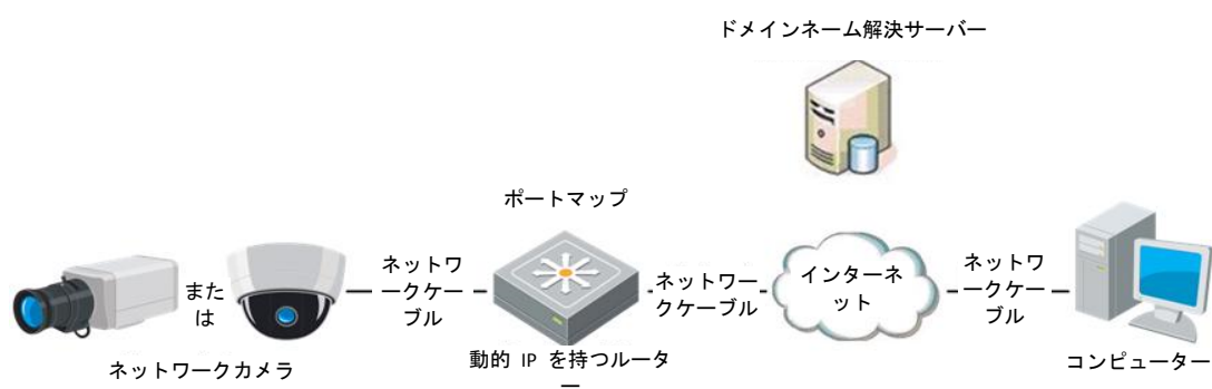
図 2-7 通常のドメイン名称の解決
