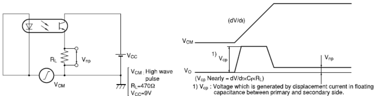
Fig.17 同相除去電圧の測定回路
