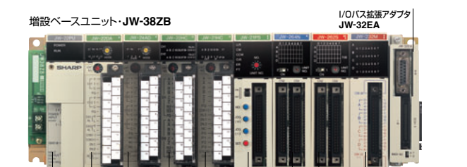
増設ベースユニット・JW-38ZB アナログ出力ユニット JW-22DA 高速カウンタユニット JW-22HC パルス出力ユニット JW-21PS 64点出力ユニット JW-262S 電源ユニット JW-22PU アナログ入力ユニット JW-24AD 高速カウンタユニット JW-21HC 64点入力ユニット JW-264N 32点出力ユニット JW-232M
