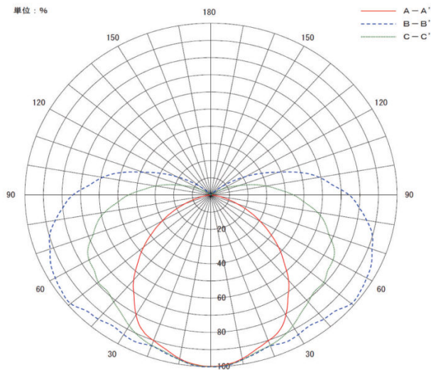
【鉛直配光曲線図】
