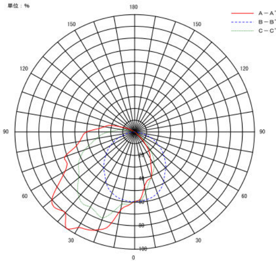
【鉛直配光曲線図】
