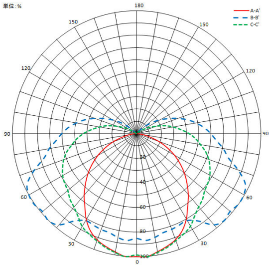
【鉛直配光曲線図】
