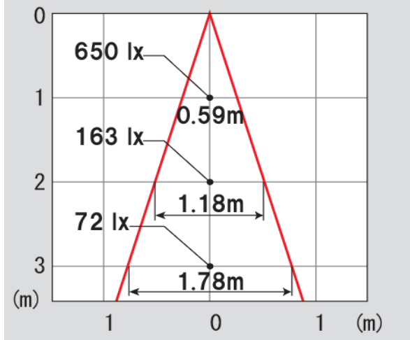
水平面照度 [lx] Ra94・33°
