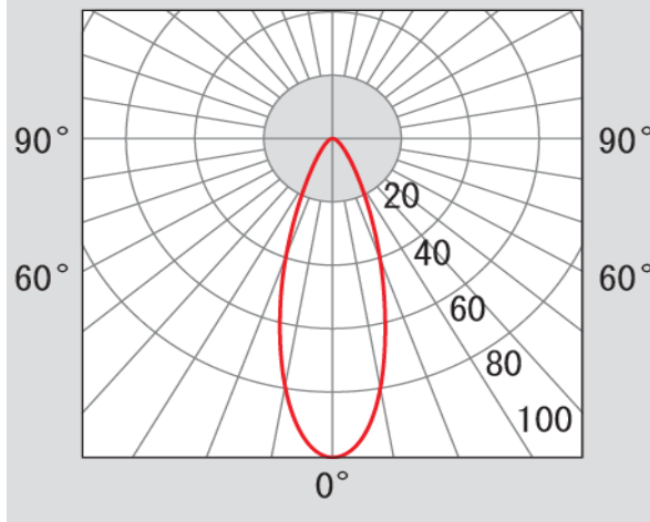
配光曲線 [%] Ra94・33°
