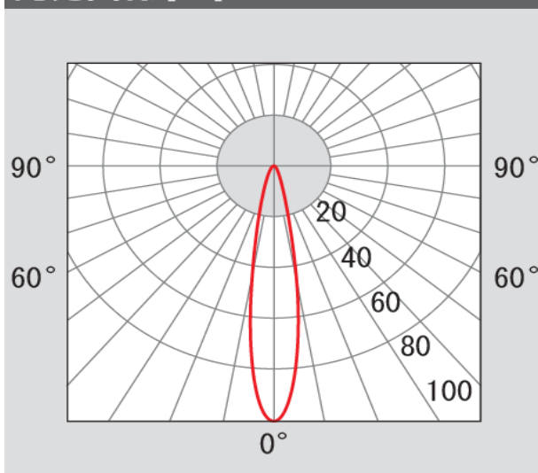
配光曲線 [%] Ra84・20°
