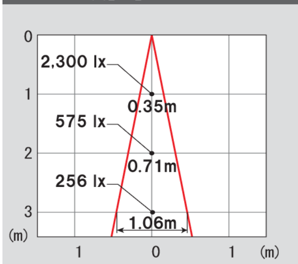
水平面照度 [lx] Ra84・20°
