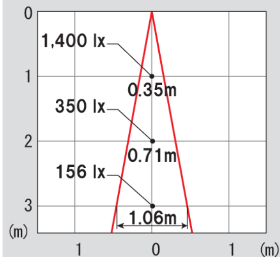
水平面照度 [lx] Ra94・20°
