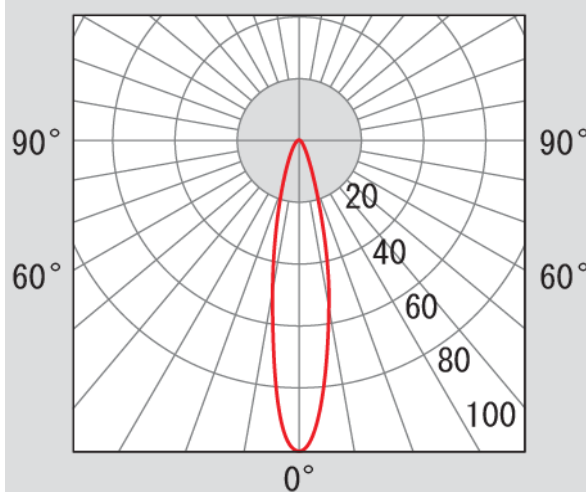
水平面照度 [lx] Ra94・20°
