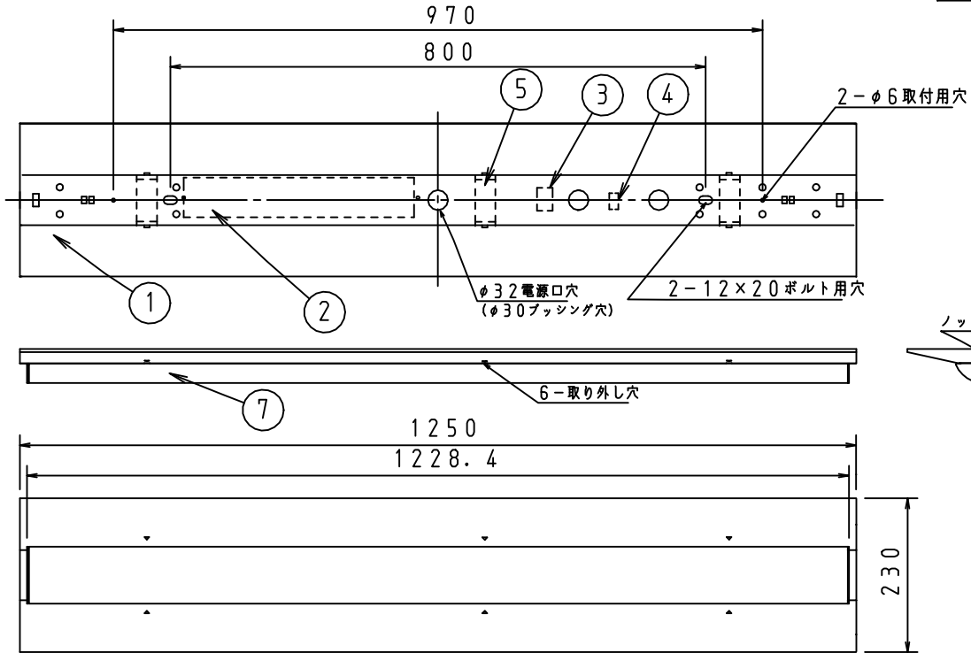
側面詳細図
