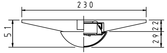
側面詳細図
