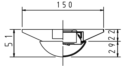
側面詳細図
