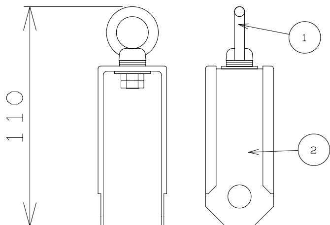
取り付け金具
