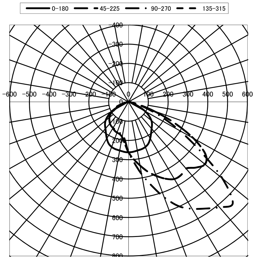
配光曲線(cd/1,000Lm)
