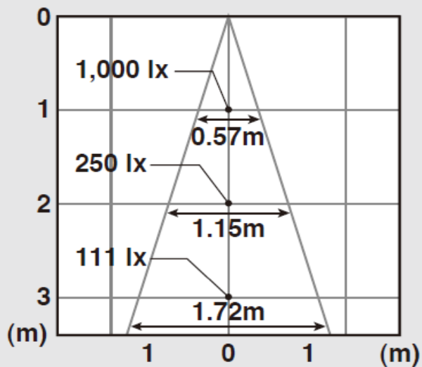
水平面照度[lx] Ra85・32°
