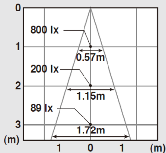
水平面照度[lx] Ra95・32°
