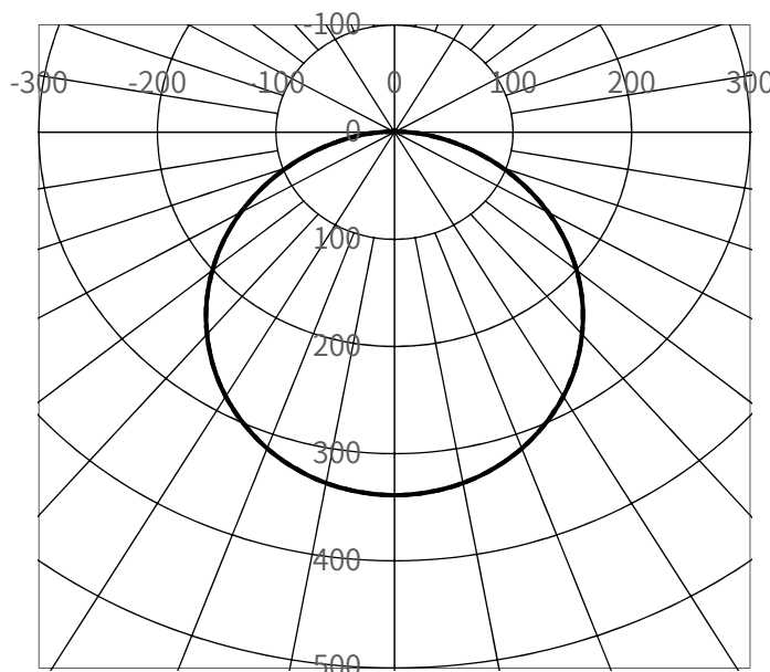
配光曲線(cd/1,000Lm)
