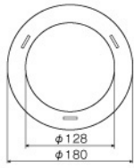
リングフレーム (鋼板)
