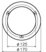
アジャストプレート (鋼板・焼付塗装)
