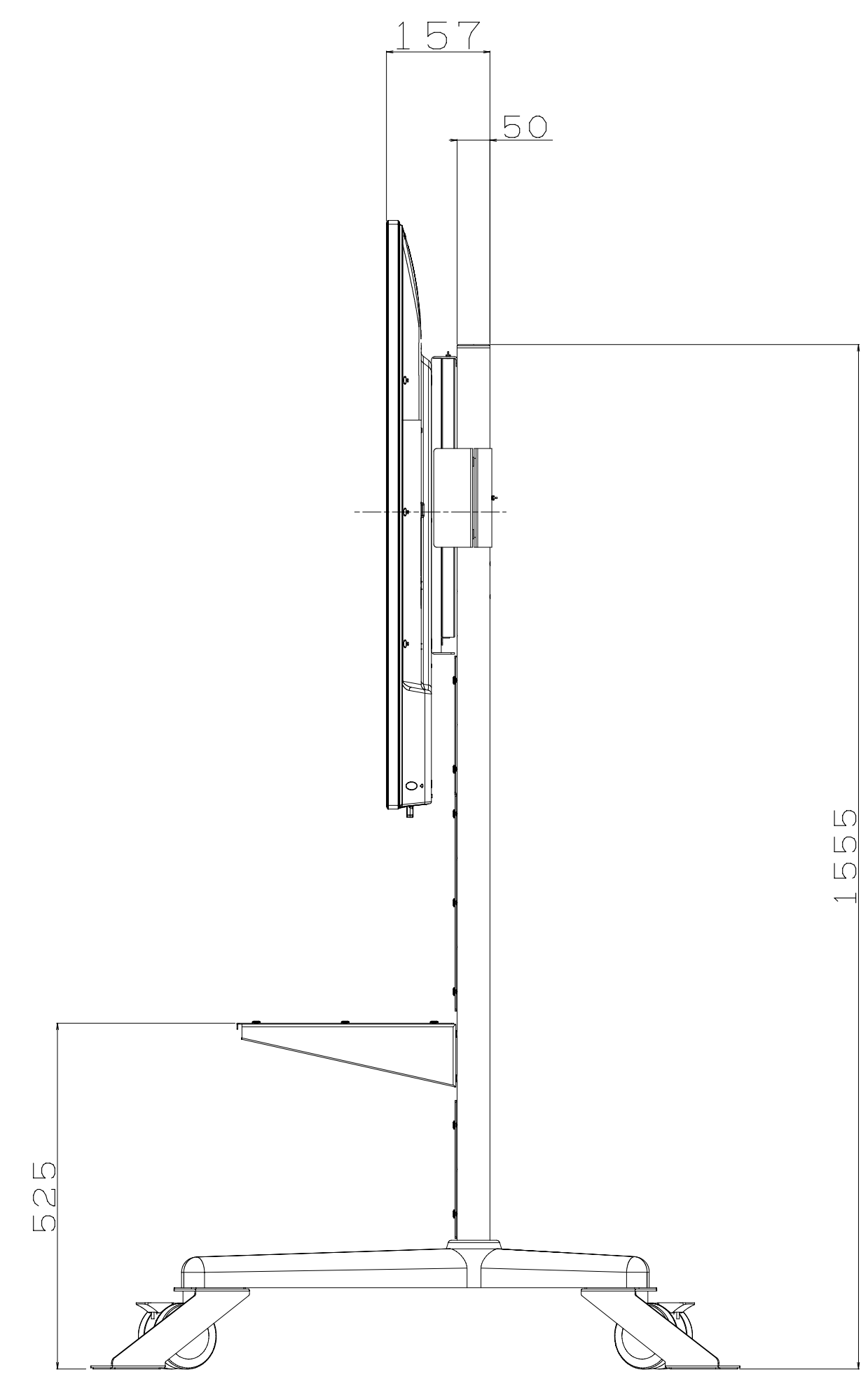
フロアスタンド (PN-H701 横取付時) PN-ZS601 外観図
