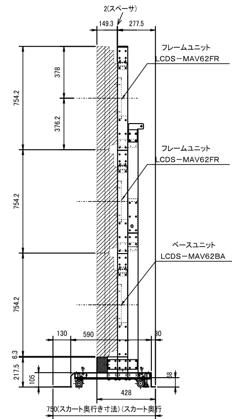
マルチディスプレイフロアスタンド (横取付3段3列)
