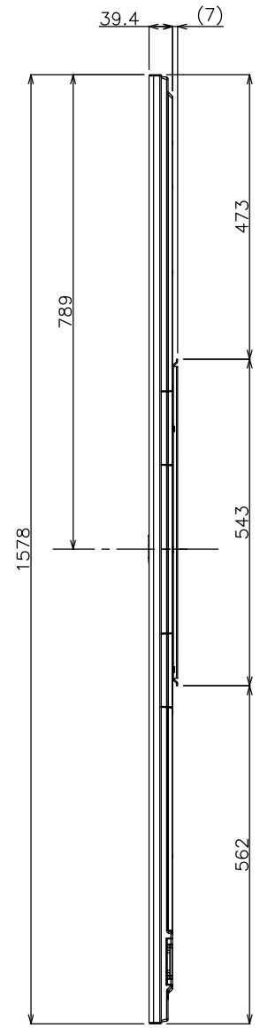
壁掛け金具 (PN-R703 縦取付時) PN-ZK703 外観図
