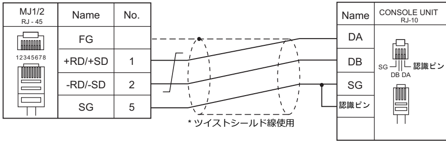
結線図 3 - M4
