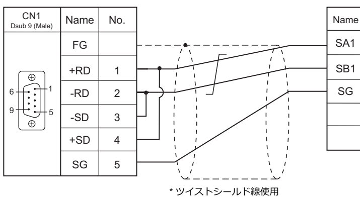
結線図 3 - C4
