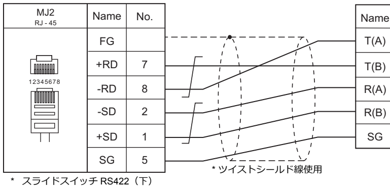
結線図 5 - M4
