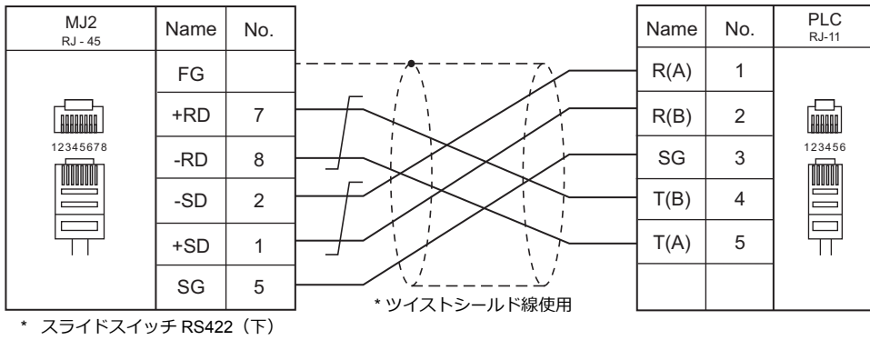
結線図 4 - M4
