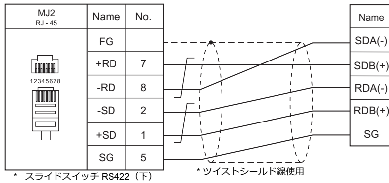
結線図 2 - M4
