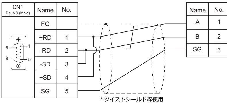
結線図 1 - C4
