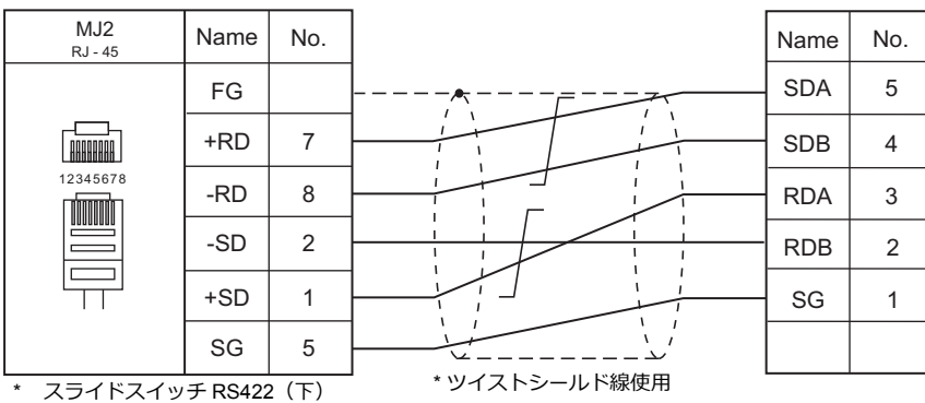
結線図 6 - M4
