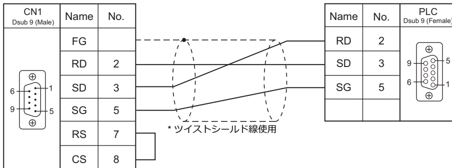
結線図 2 - C2
