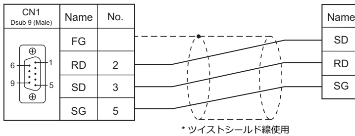
結線図 1 - C2
