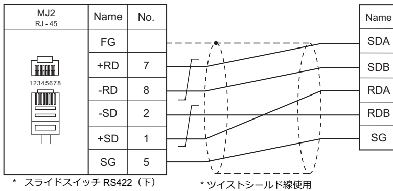
結線図 4 - M4
