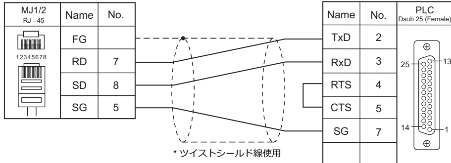
結線図 1 - M2
