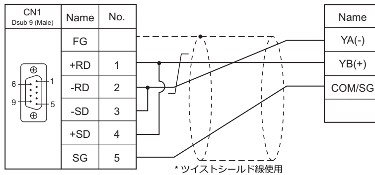
結線図 1 - C4
