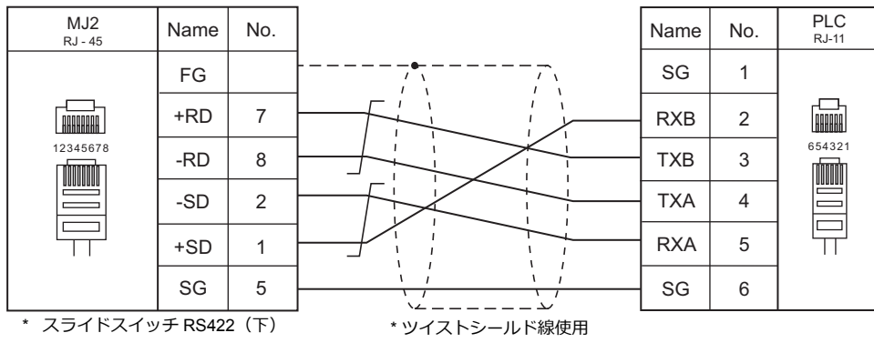
結線図 4 - M4
