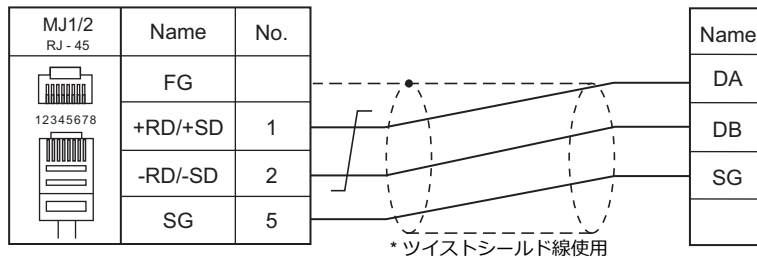
結線図 1 - M4
