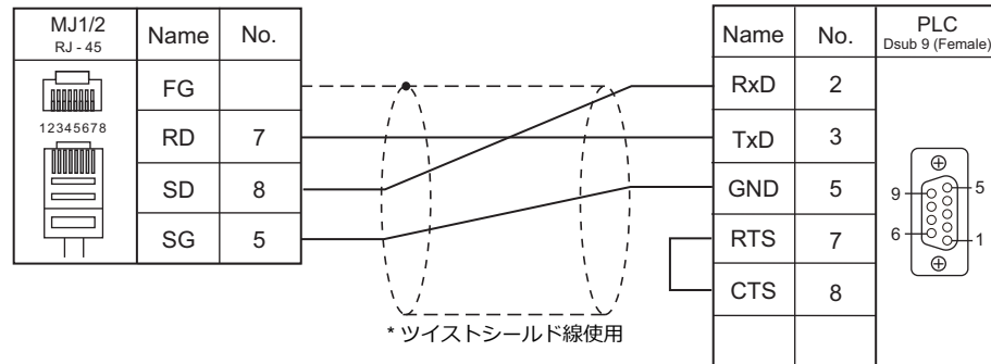
結線図 3 - M2
