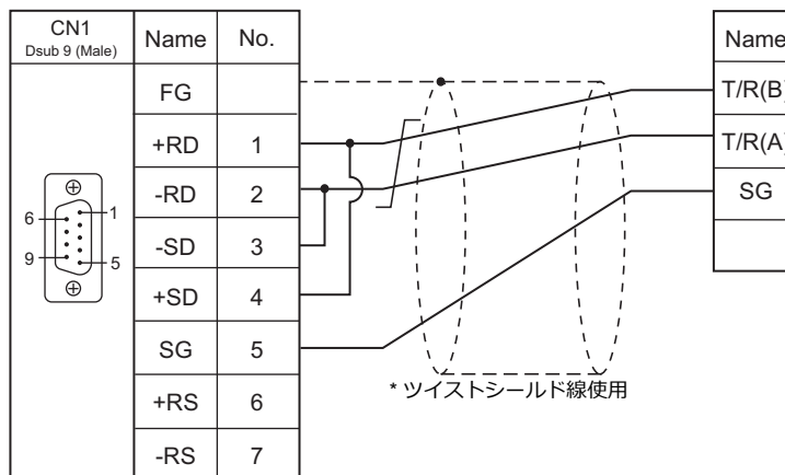
結線図 1 - C4
