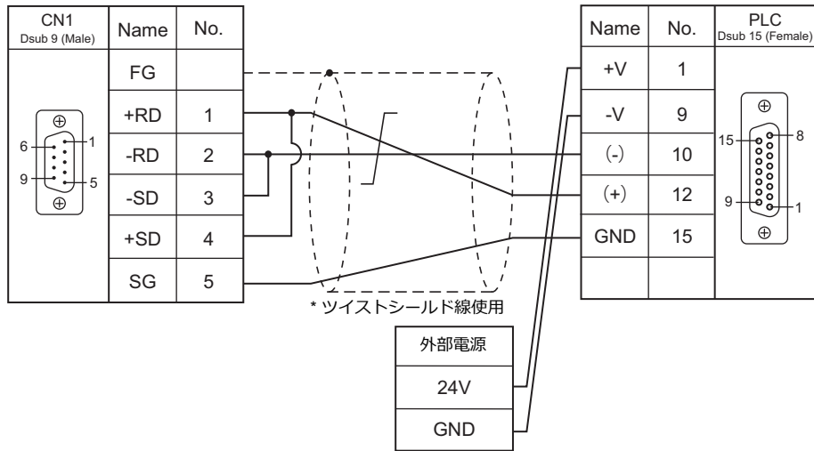
結線図 1 - C4
