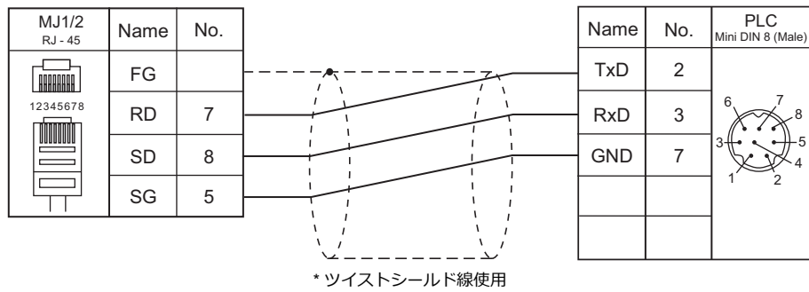
結線図 2 - M2
