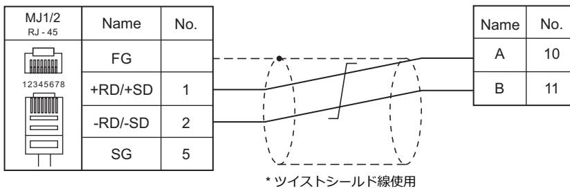
結線図 7 - M4
