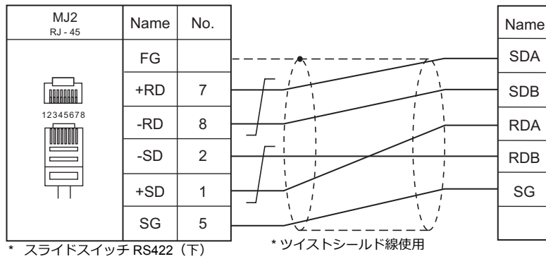
結線図 5 - M4
