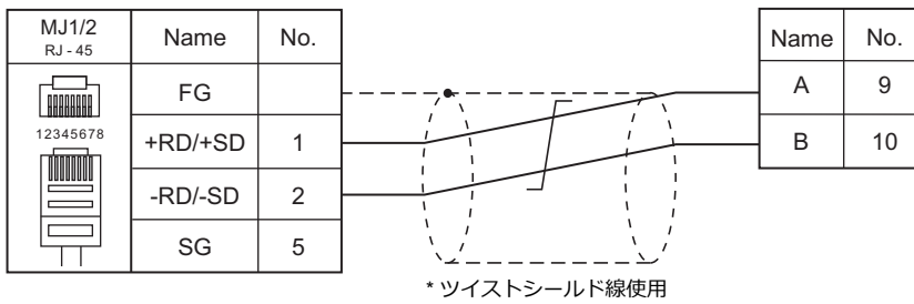
結線図 5 - M4
