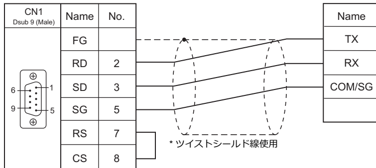
結線図 1 - C2
