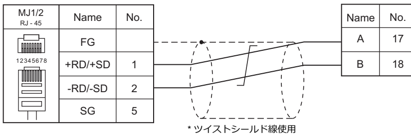
結線図 4 - M4
