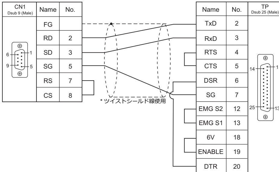
結線図 2 - C2
