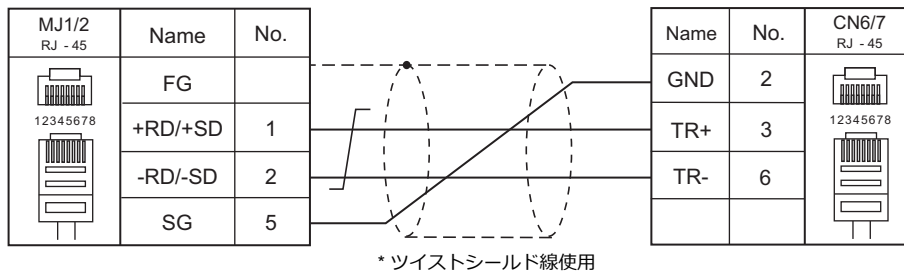
結線図 1 - M4
