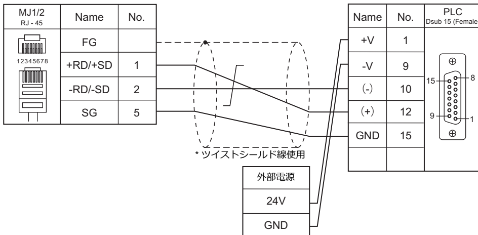
結線図 1 - M4
