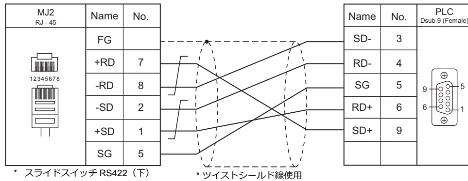
結線図 3 - M4
