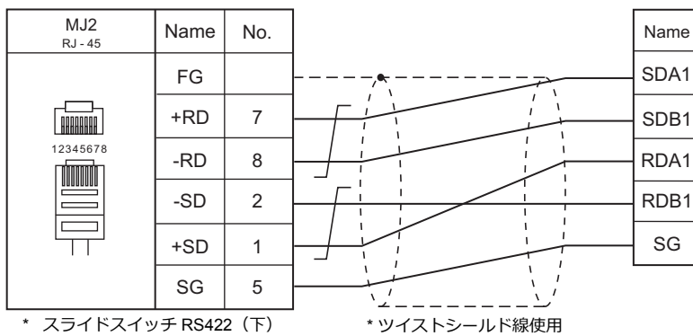
結線図 5 - M4
