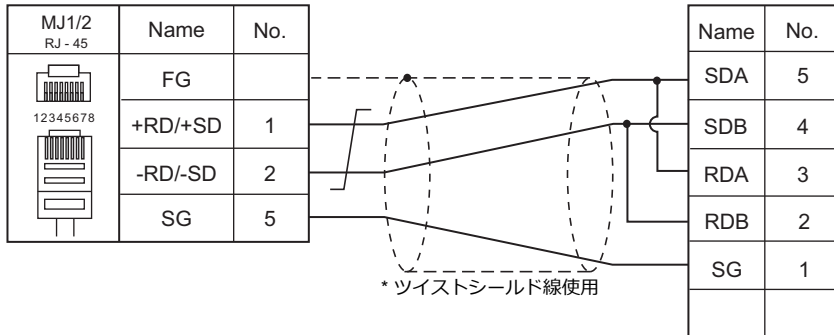
結線図 4 - M4
