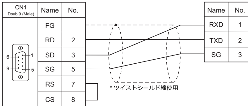
結線図 1 - C2
