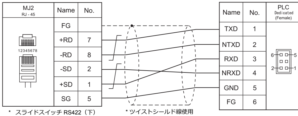
結線図 1 - M4
