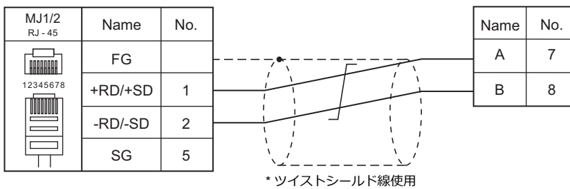
結線図 6 - M4
