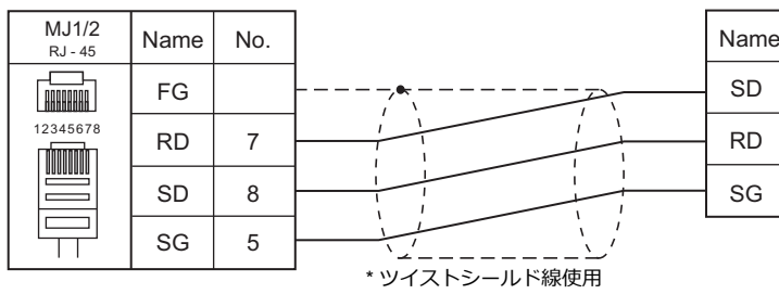
結線図 1 - M2
