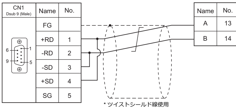
結線図 2 - C4
