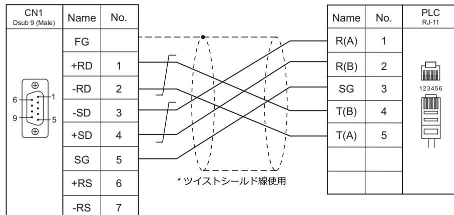
結線図 2 - C4
