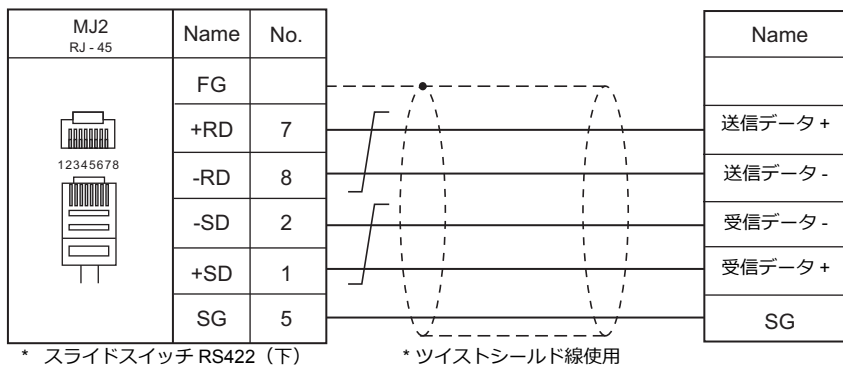
結線図 2 - M4
