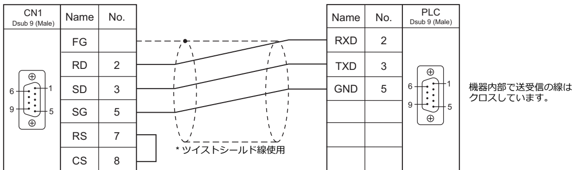
結線図 1 - C2
